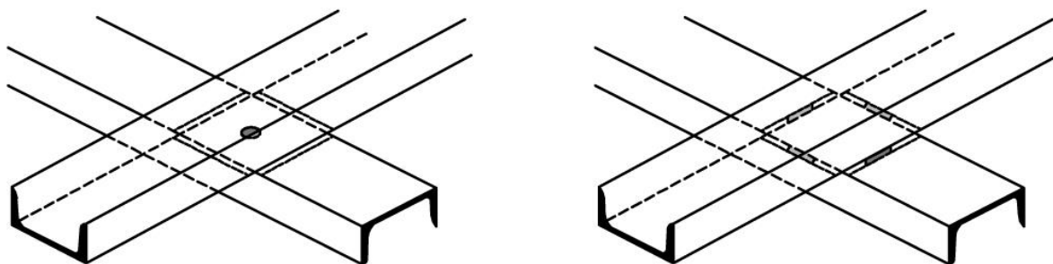
Рисунок А.3 – Примеры выполнения металлоконструкций с соединениями элементов внахлестку (сварные швы выполняются прерывистыми или с пробивкой отверстий для исключения взрыва)
