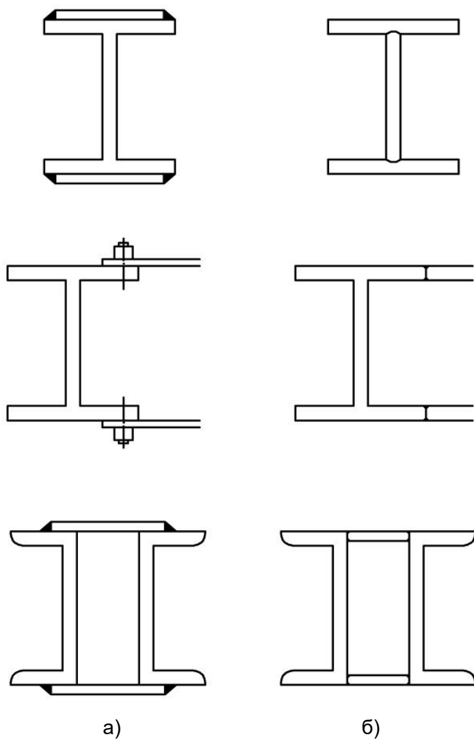
Рисунок А.7 – Примеры выполнения технологических отверстий для выхода цинка и газов в металлоконструкциях с наличием опорной плиты
