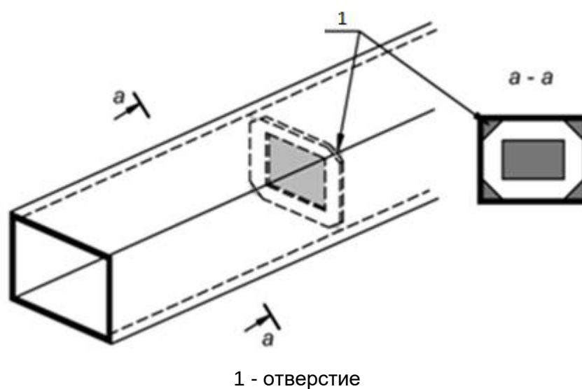
Рисунок А.4 – Пример выполнения внутренней перегородки в пустом профиле (перегородка выполняется с вырезами по углам)
